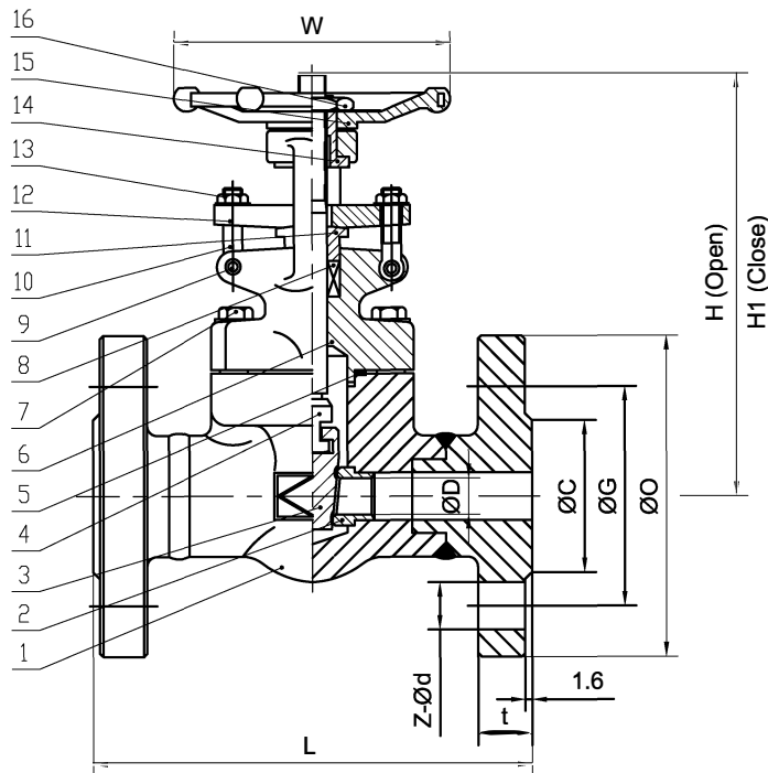
NPS DN L D C G O t Z-Ød W H H 1 1/2" 15 108 10.5 35 67 89 10 4-Ø14 100 151 138 3/4" 20 117 13.0 43 73 98 11 4-Ø14 100 158 142 1" 25 127 17.5 51 83 108 12 4-Ø14 125 190 170 1 1/4" 32 140 23.0 64 87 117 13 4-Ø14 160 217 190
